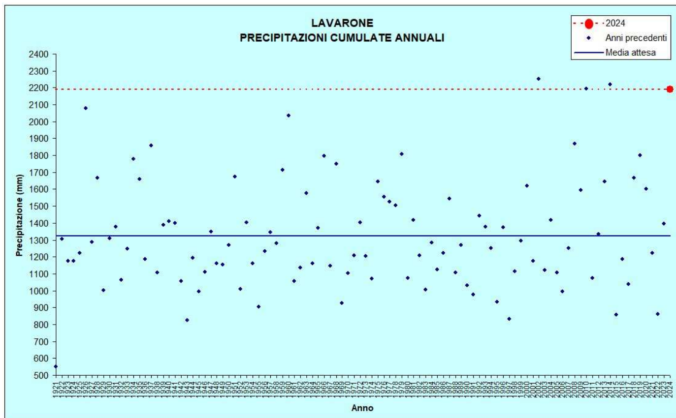
Figura 8: Precipitazioni annuali
