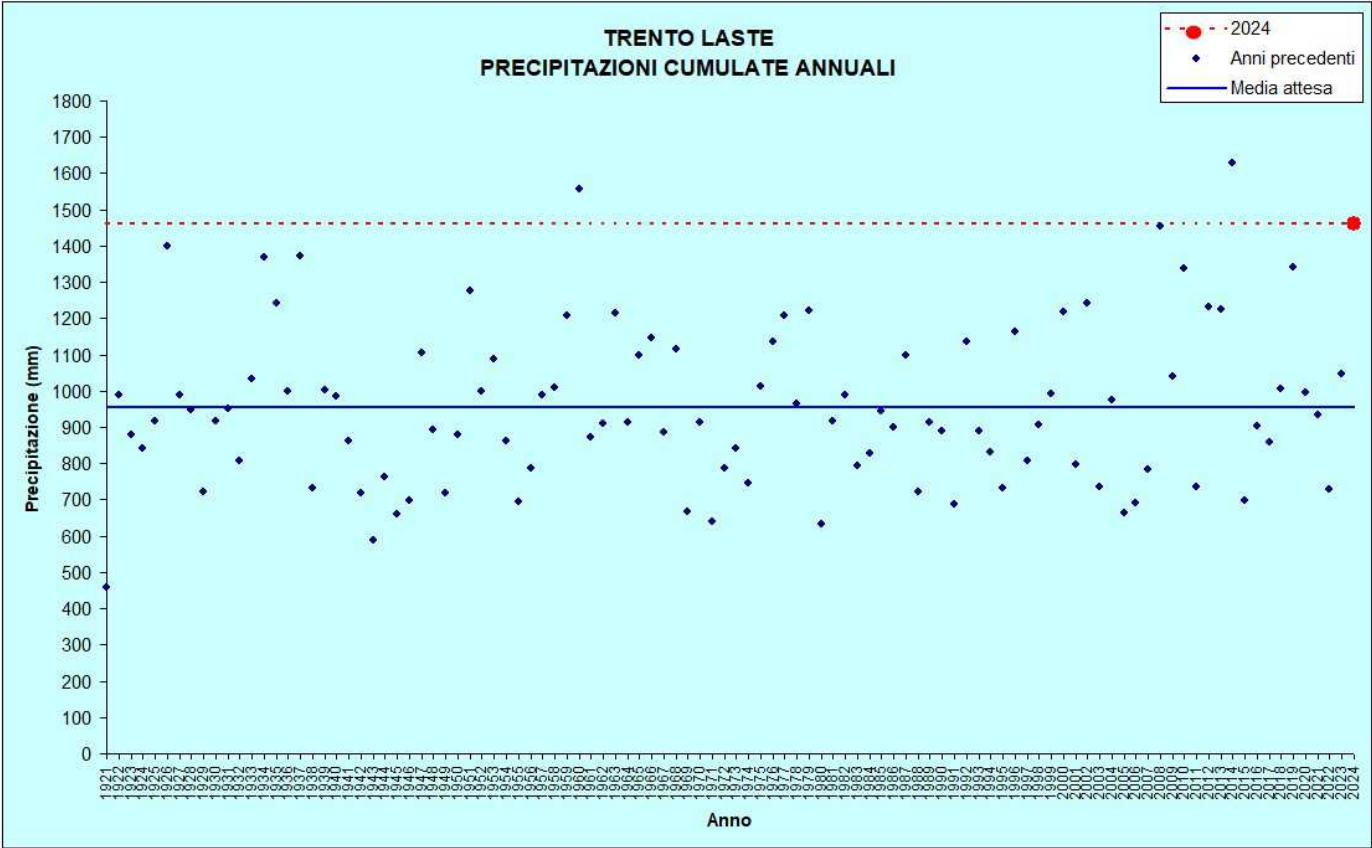
Figura 4: Precipitazioni annuali
