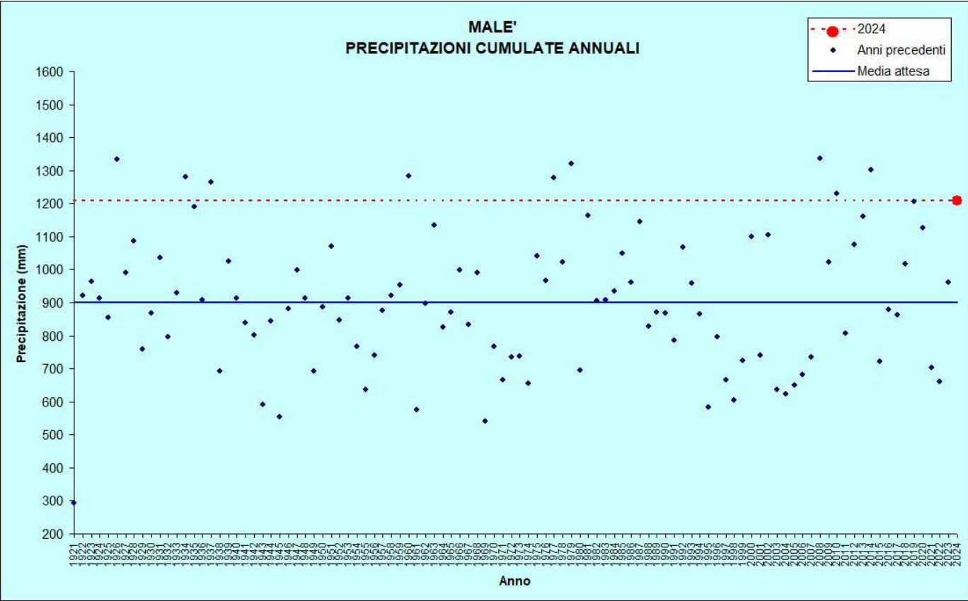
Figura 10: Precipitazioni annuali
