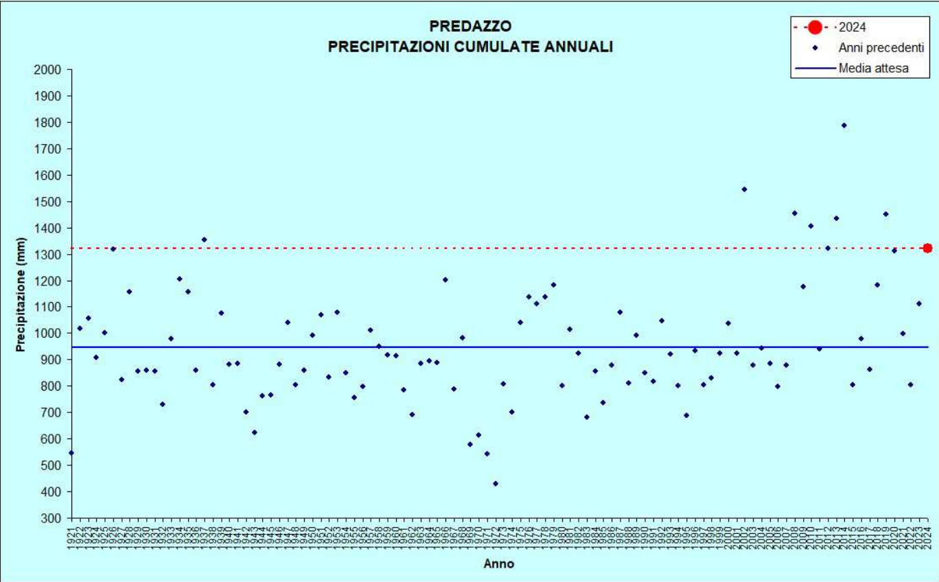
Figura 18: Precipitazioni annuali
