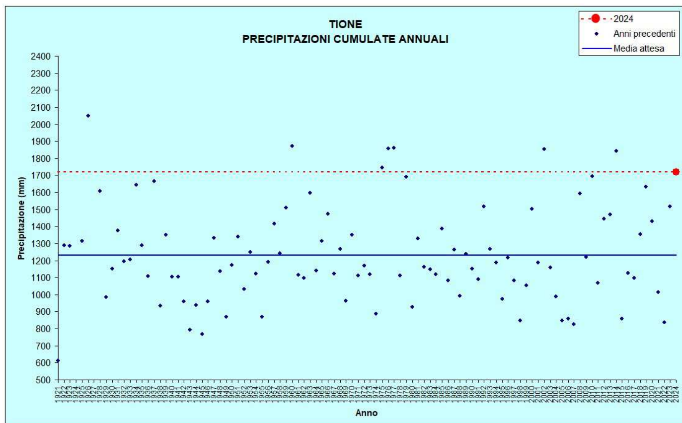
Figura 12: Precipitazioni annuali
