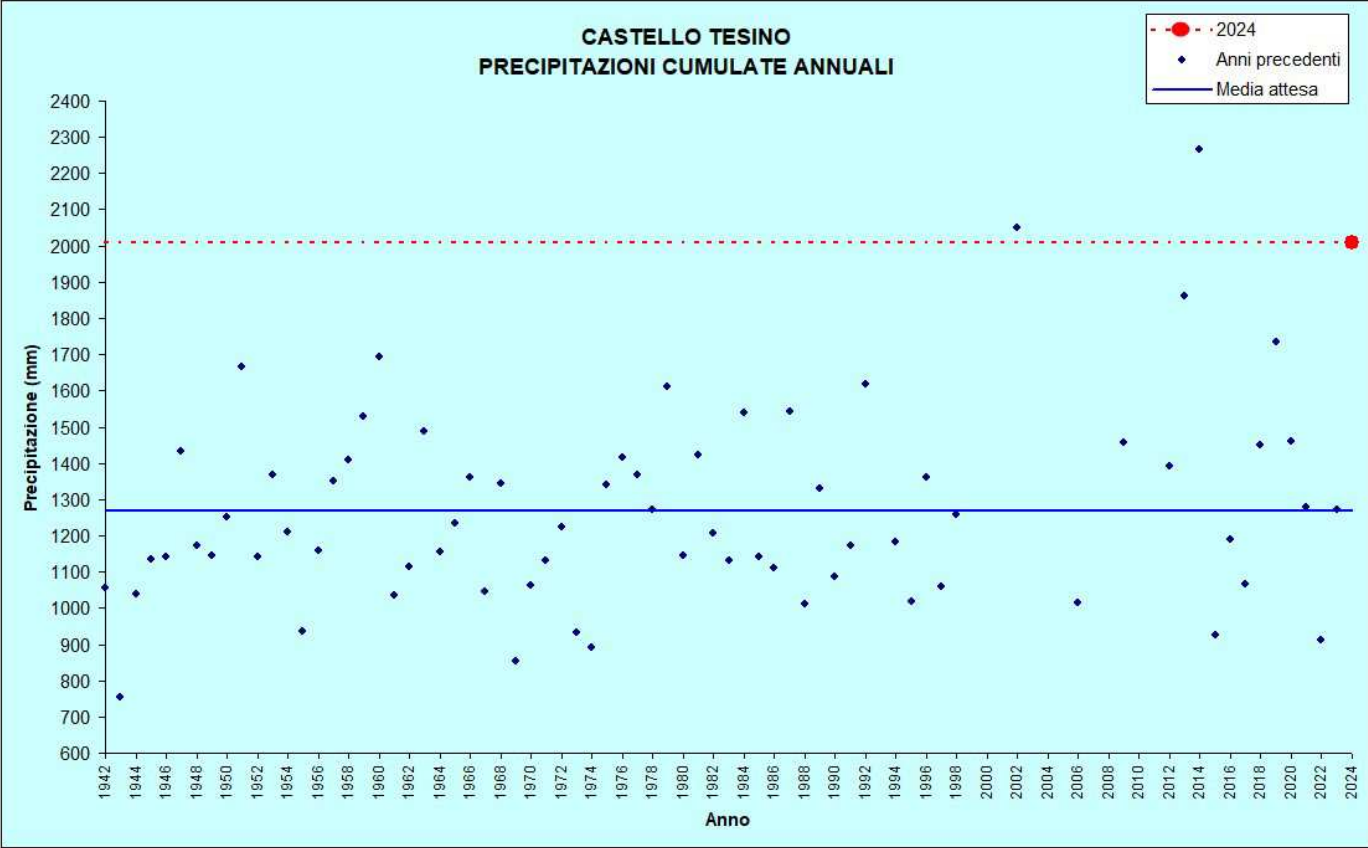
Figura 6: Precipitazioni annuali
