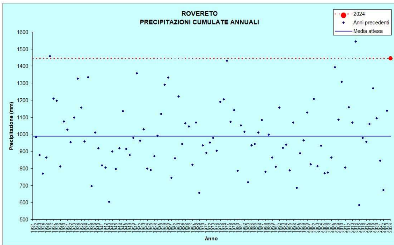
Figura 16: Precipitazioni annuali
