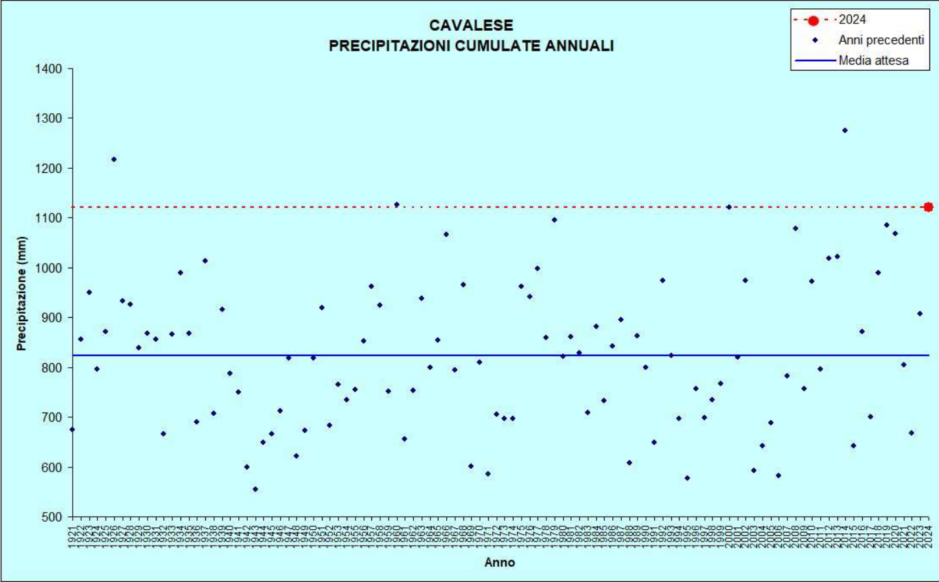
Figura 14: Precipitazioni annuali
